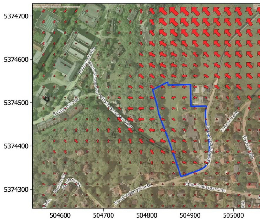
Abb. 11: Kaltluftströmung ca. 30 Minuten nach Beginn einer Kaltluftsituation (aus: Nielinger & Hasel (2021))
