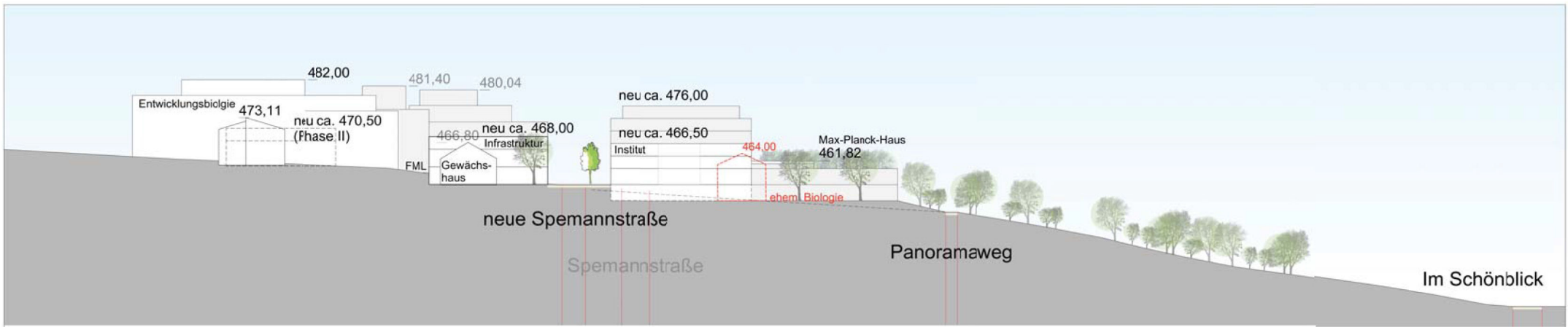
Schnitt A - A Phase I
