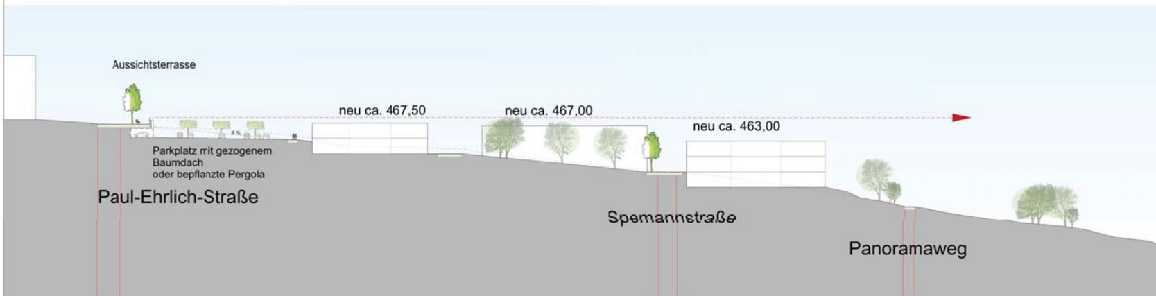
Schnitt C - C Phase II
