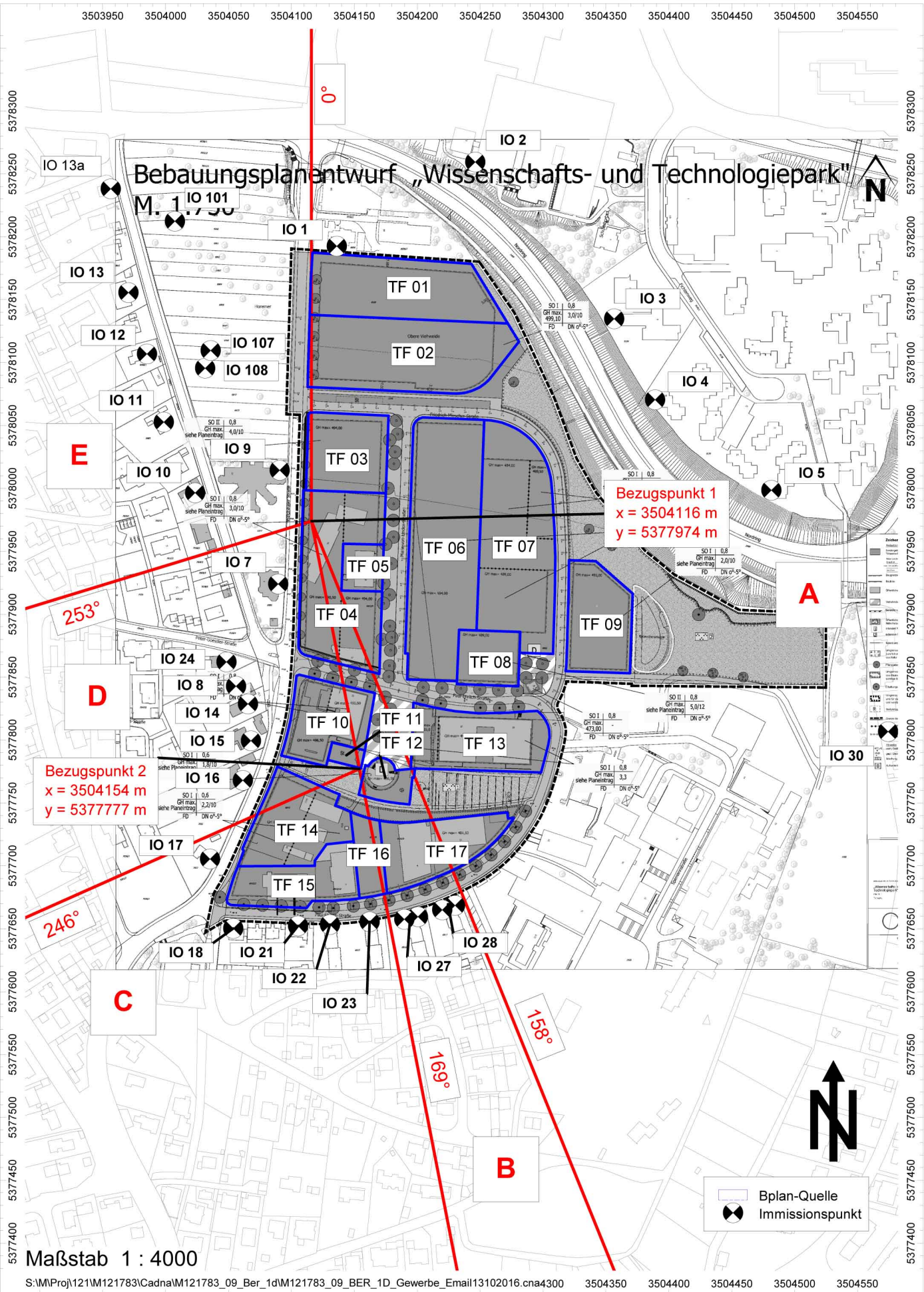
Plan 1: Plan zur Festsetzung der Emissionskontingente (Teilflächen und Richtungssektoren)
