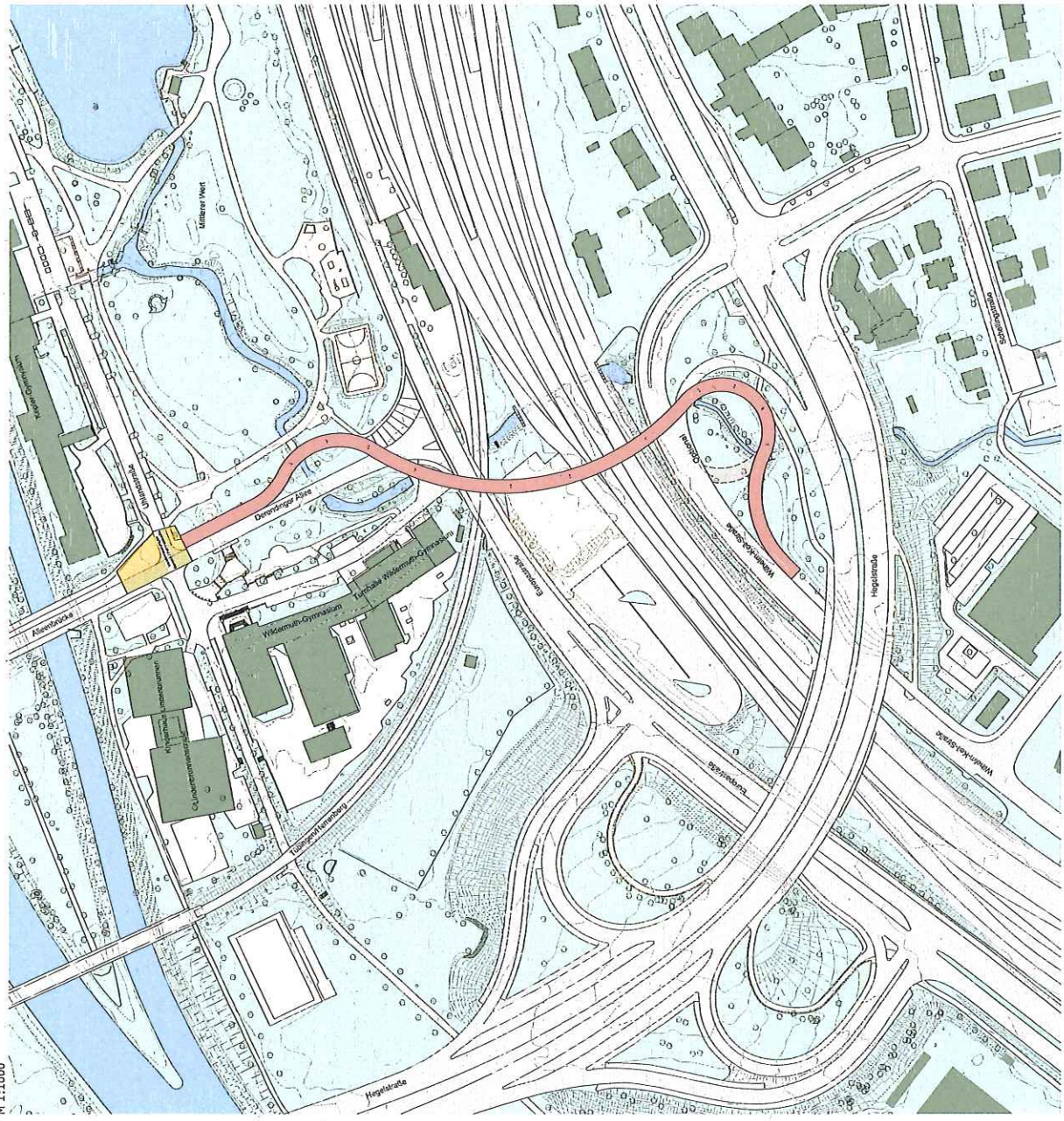
Radwegbrücke - Querung West Lageplan Brückenverbreiterung M 1:1000
