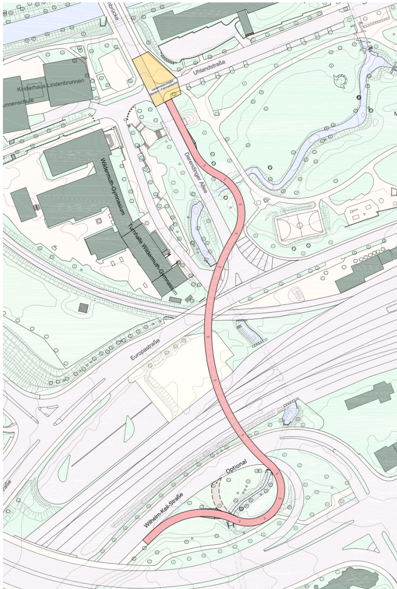
Lageplan Radwegbrücke lichte Breite 4,0 m
