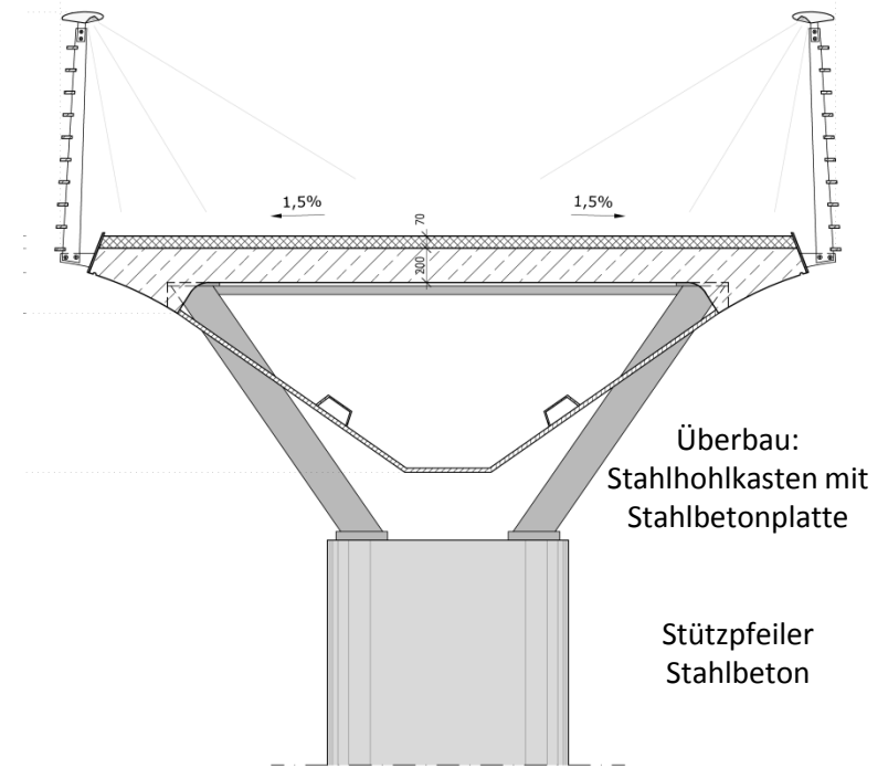
Querschnitt Radwegbrücke lichte Breite 4,0 m
