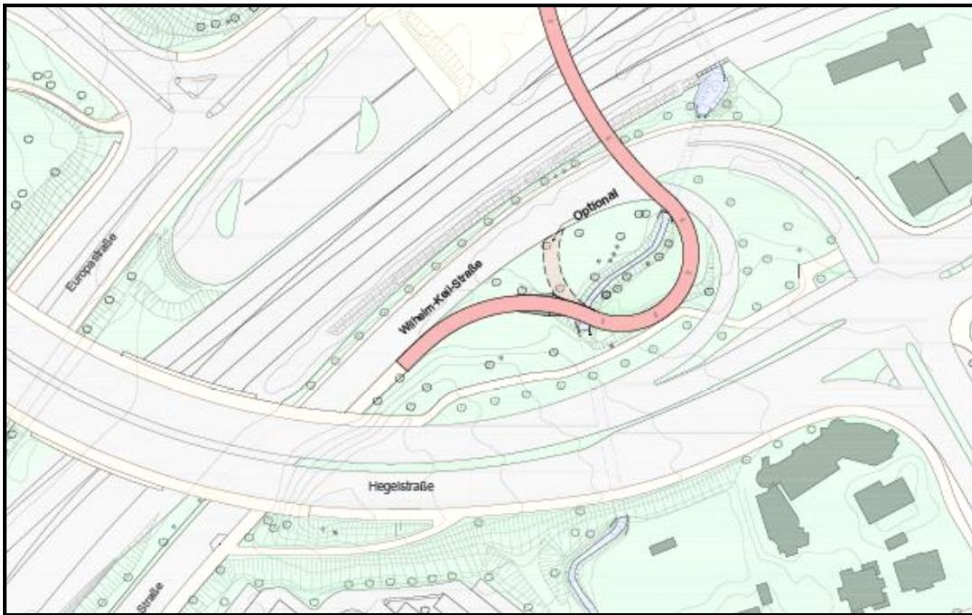
Entwurf Sobek und tragwerke+ zur Rampenführung in der Wilhelm-Keil-Straße
