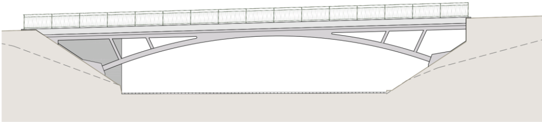
Variante 1: Aufgeständerte Bogenbrücke aus Stahl- und Spannbeton Bruttobaukosten 3,5 Mio €
