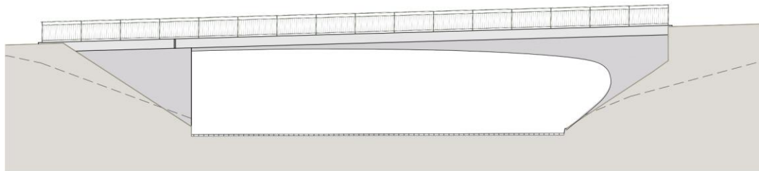
Variante 4: Einhüftiger Rahmen aus Spannbeton Bruttobaukosten 2,15 Mio €
