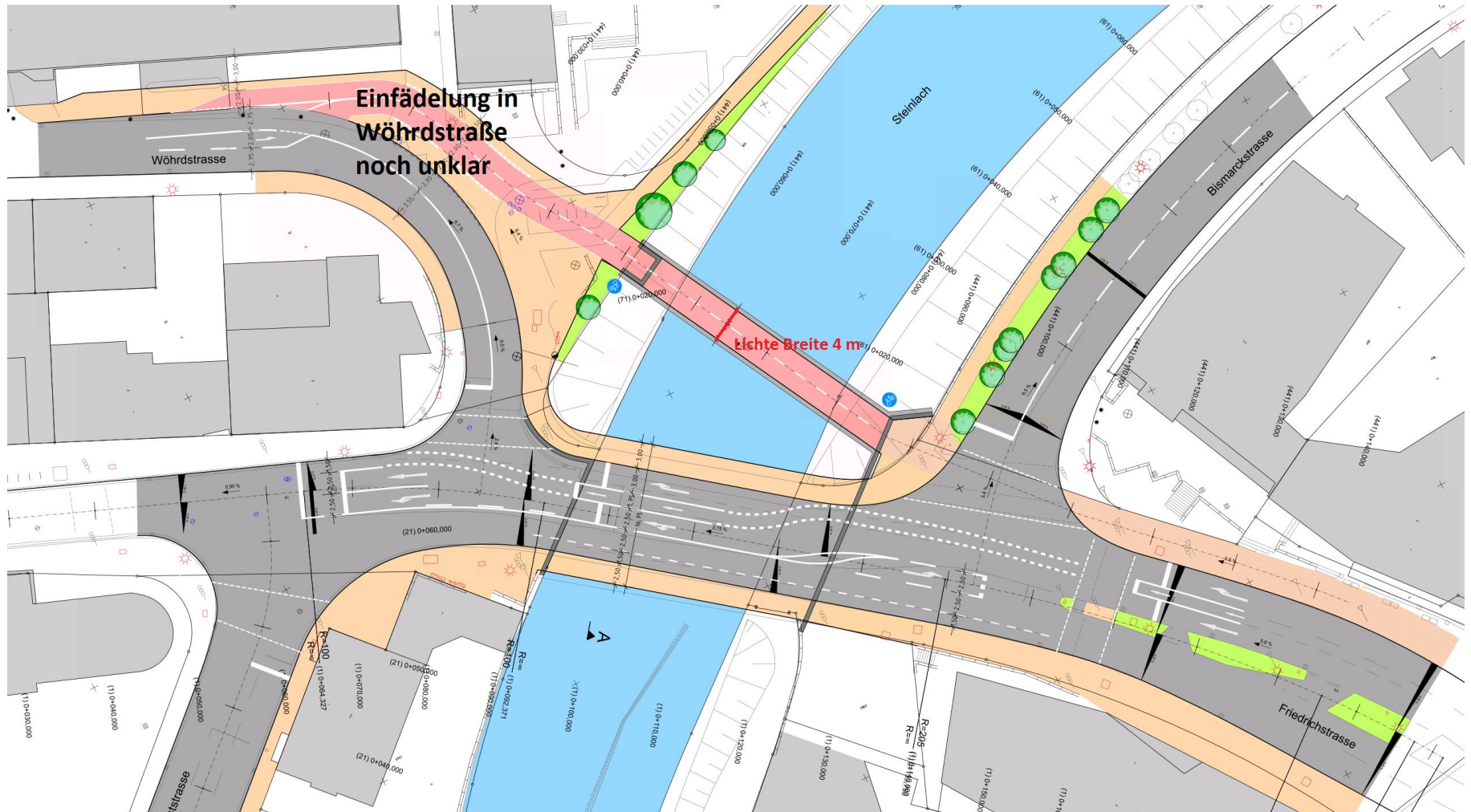
Lageplan beider Steinlachbrücken – Planungsstand Januar 2019: Straßenbrücke Friedrichstraße und Radwegbrücke Wöhrdstraße
