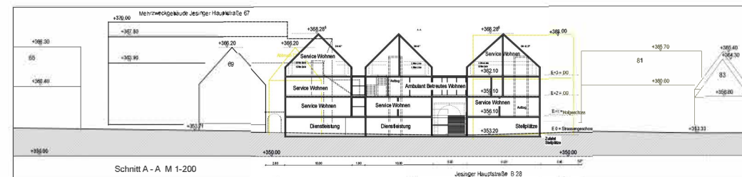
Schnitt A - A M 1-200
