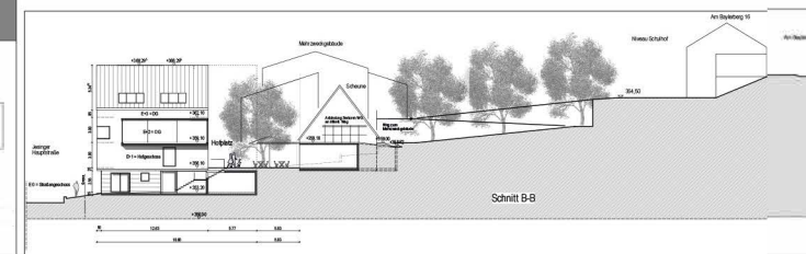
Schnitt B - B M 1-200
