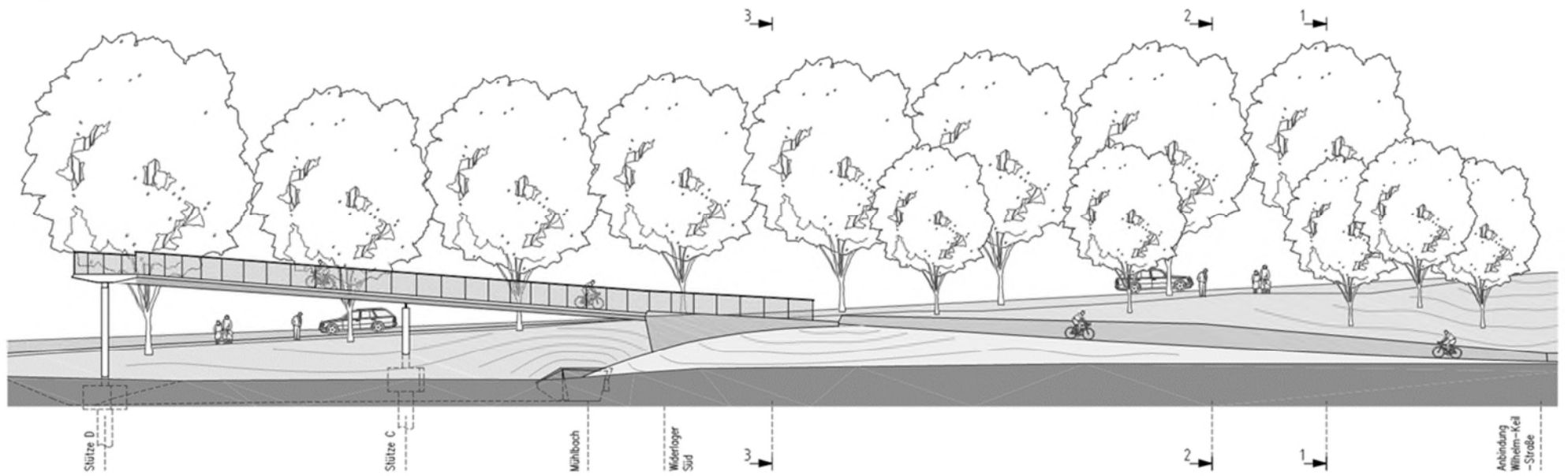
Ansicht Rampe Süd A-A M 1: 100
