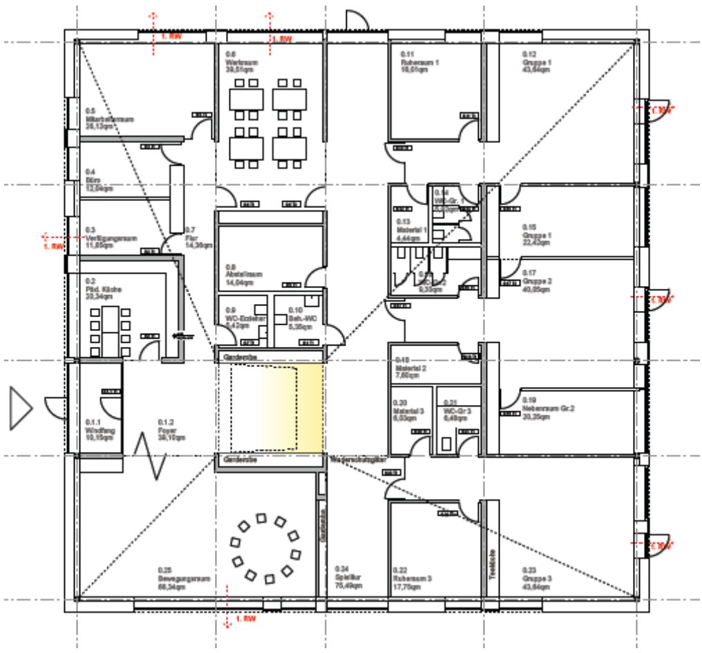
Grundriss Kinderhaus
