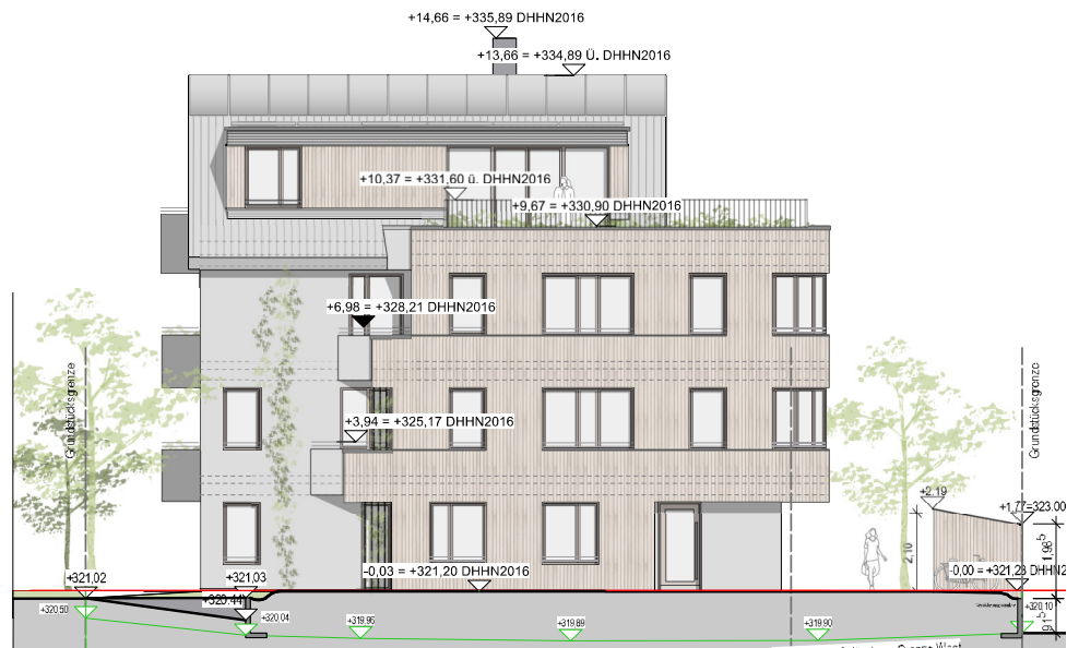
Haus 1 Südansicht
