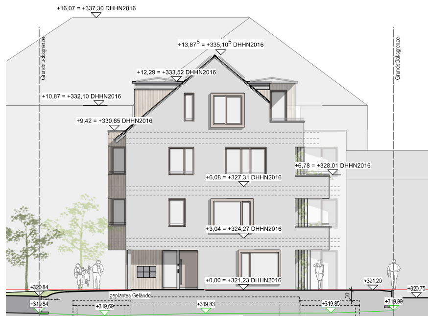
Haus 2 Nordansicht
