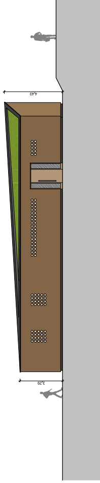
Ansicht Nord-Ost M.1:100
