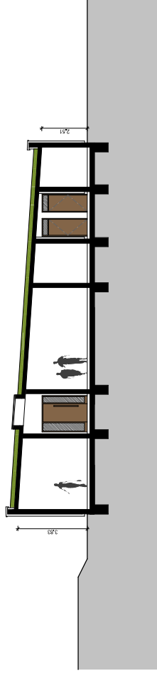
Schnitt A-A M.1:100
