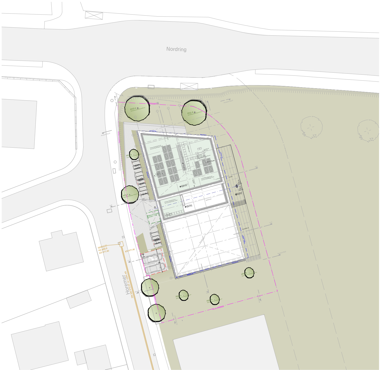
Lageplan 1:1500
