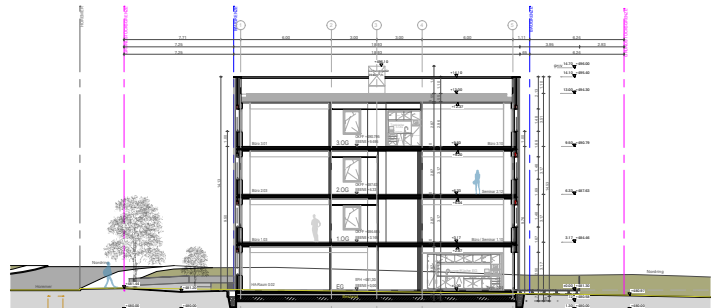
Schnitt B-B 1:1500
