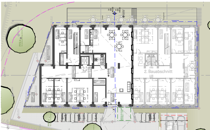
Grundriss EG 11500
