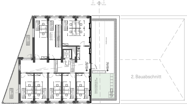
Grundriss 3.OG 11500
