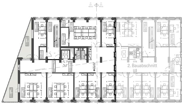
Grundriss 3.OG 11500
