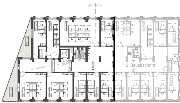
Grundriss 2.OG 11500
