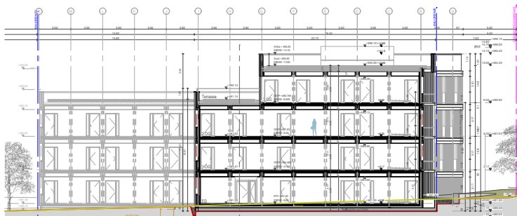
Schnitt A-A 1:1500
