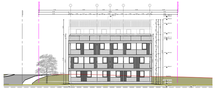
Ansicht Süd 11500
