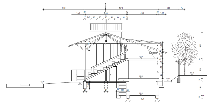
Schnitt A-A
