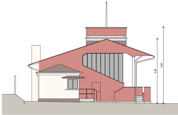
Ansicht Südost
