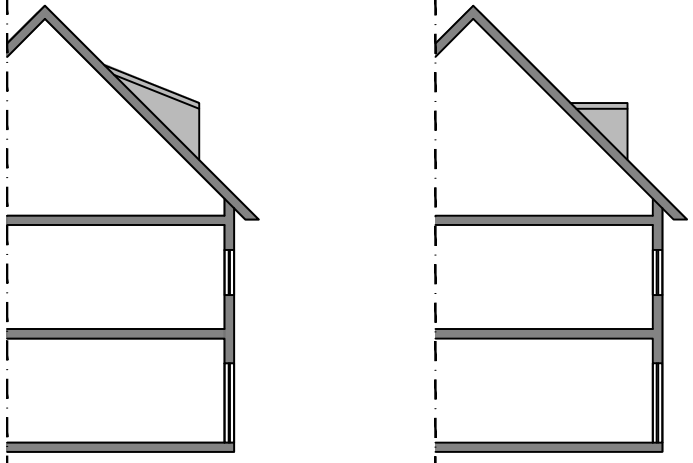
Dachneigung Gebäude über 35 °
