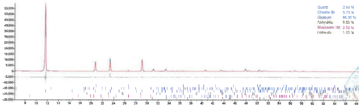
Abbildung 7: Auswertung und Schaubild der Probe 19126 B 2/24 59,50 m
