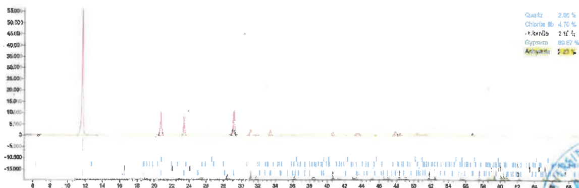
Abbildung 5: Auswertung und Schaubild der Probe B 3/24 – 67,7 m
