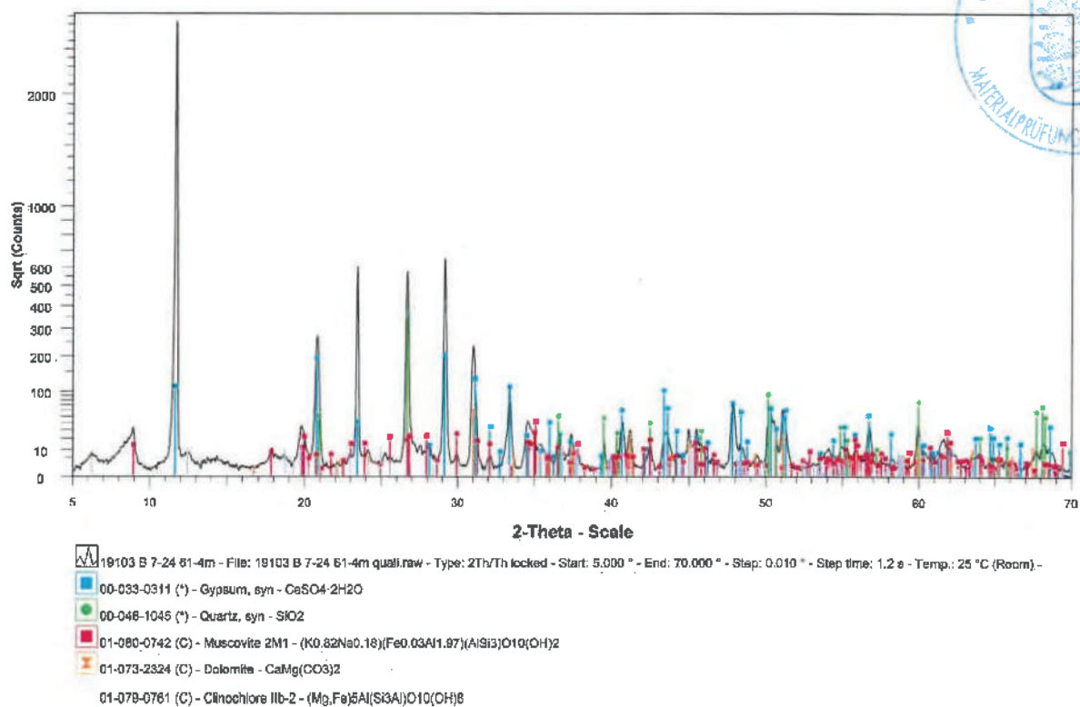
Abbildung 3: Schaubild der Probe B 7/24 – 61,4 m
