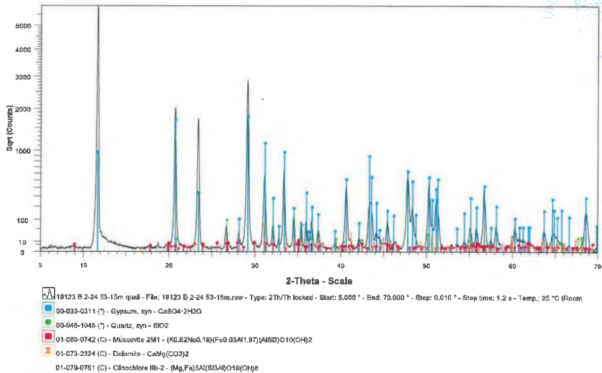
Abbildung 1: Schaubild der Probe B 2/24 – 53,15 m
