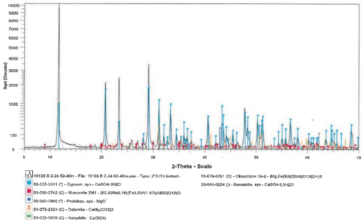
Abbildung 4: Schaubild der Probe B 2/24 – 62,40 m
