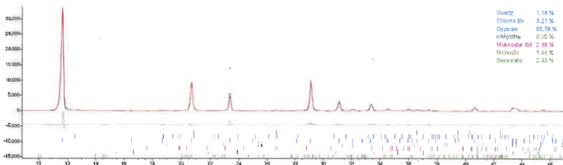
Abbildung 8: Auswertung und Schaubild der Probe 19127 B 2/24 – 61,15 m
