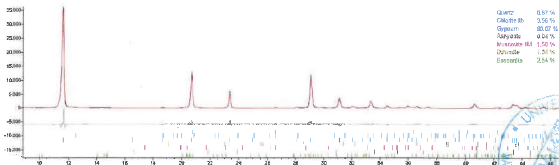
Abbildung 9: Auswertung und Schaubild der Probe 19130 B 2/24 – 75,20 m
