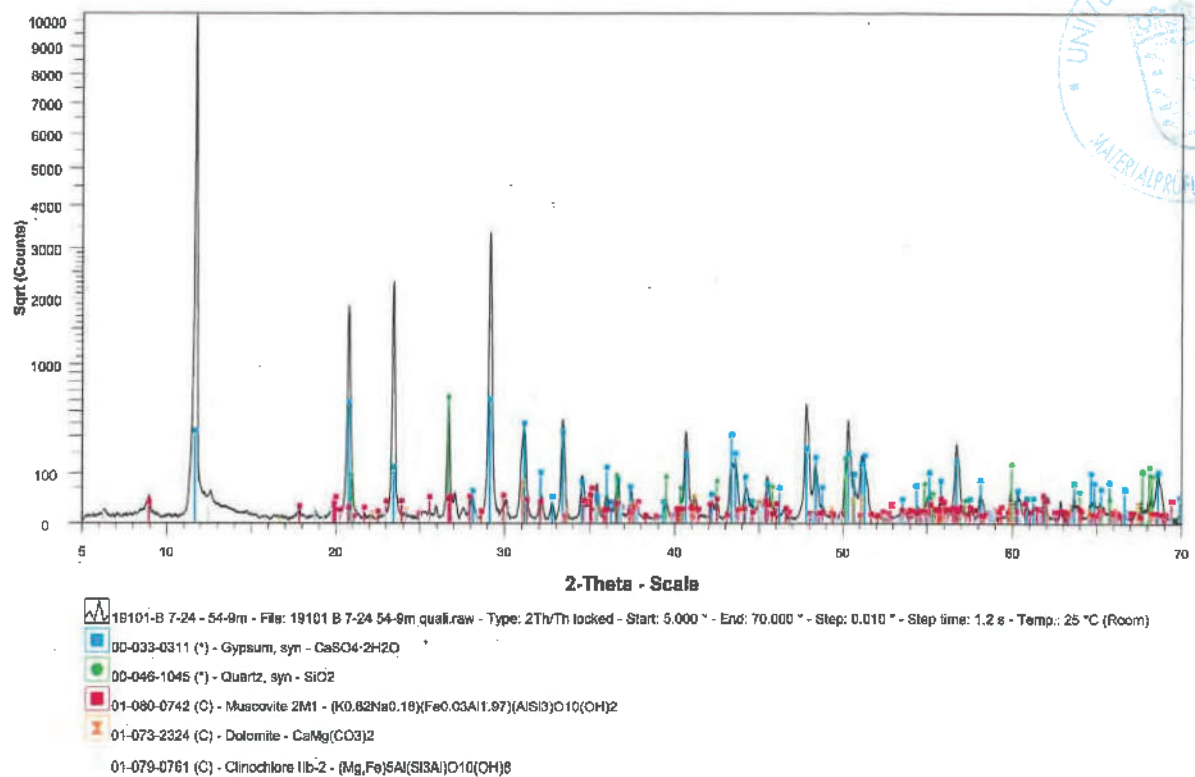
Abbildung 1: Schaubild der Probe B 7/24 – 54,9 m
