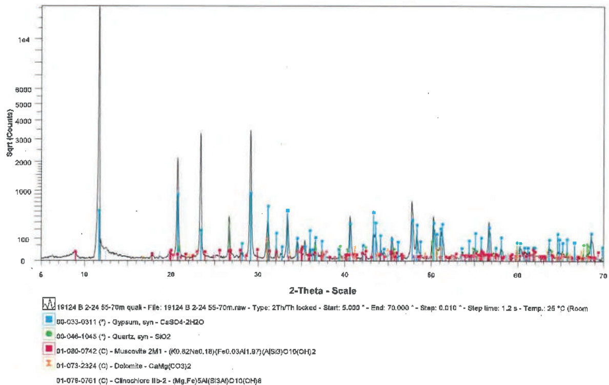
Abbildung 2: Schaubild der Probe B 2/24 – 55,70 m
