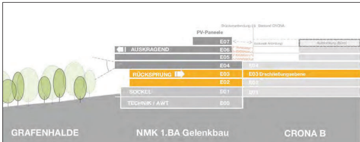
Abbildung 4: Prinzipschnitt N – S (Quelle: Machbarkeitsstudie von Heinle, Wischer und Partner vom 02.03.2021)
