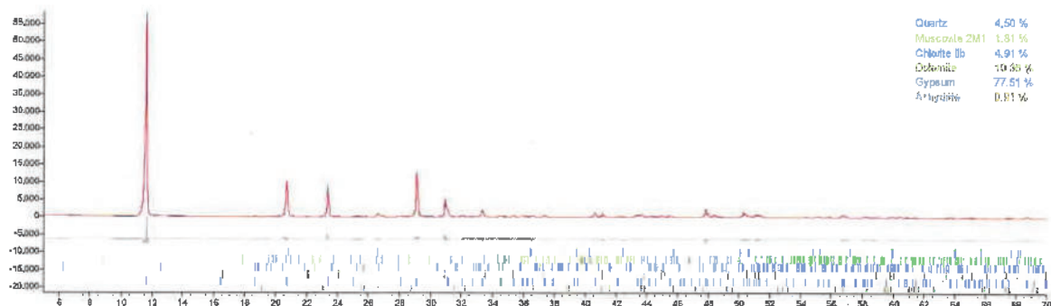
Abbildung 5: Auswertung und Schaubild der Probe 19105 B 7/24 – 62,5 m
