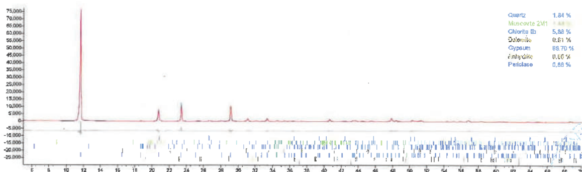
Abbildung 4: Auswertung und Schaubild der Probe 19104 B 7/24 61,9 m
