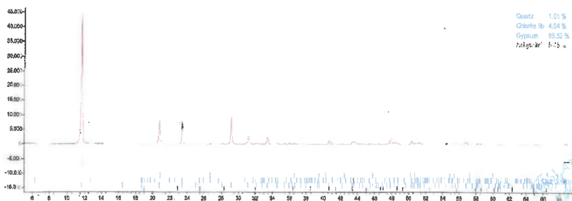
Abbildung 6: Auswertung und Schaubild der Probe B 3/24 – 68,1 m
