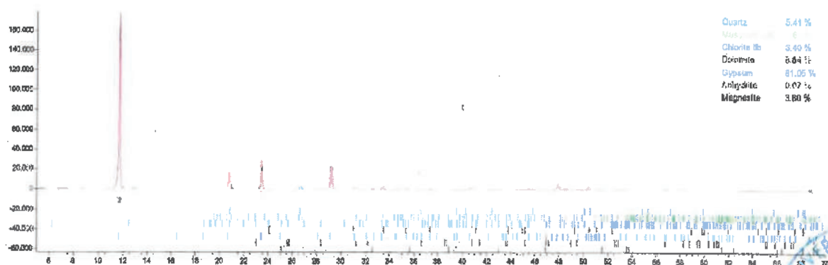
Abbildung 3: Auswertung und Schaubild der Probe B:3/24 – 63,5 m
