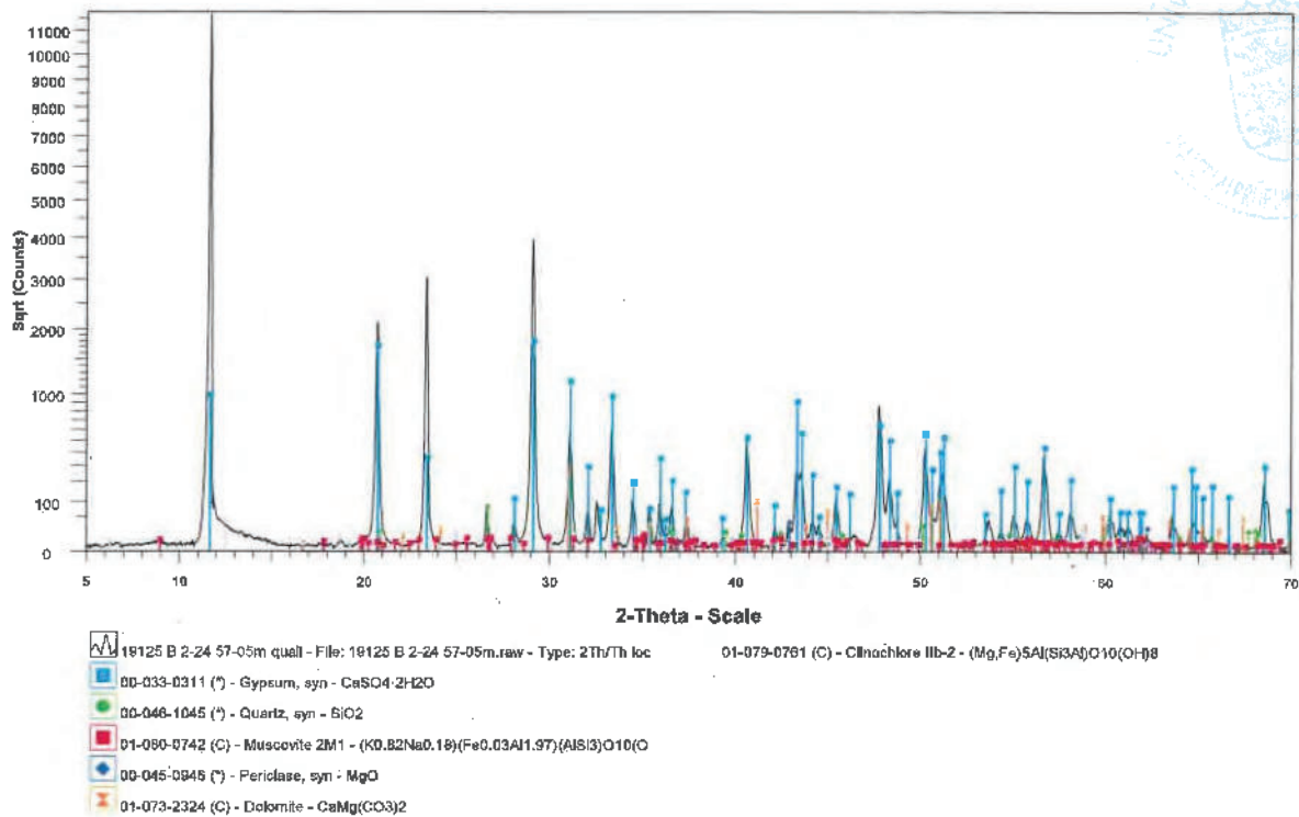
Abbildung 3: Schaubild der Probe B 2/24 – 57,05 m
