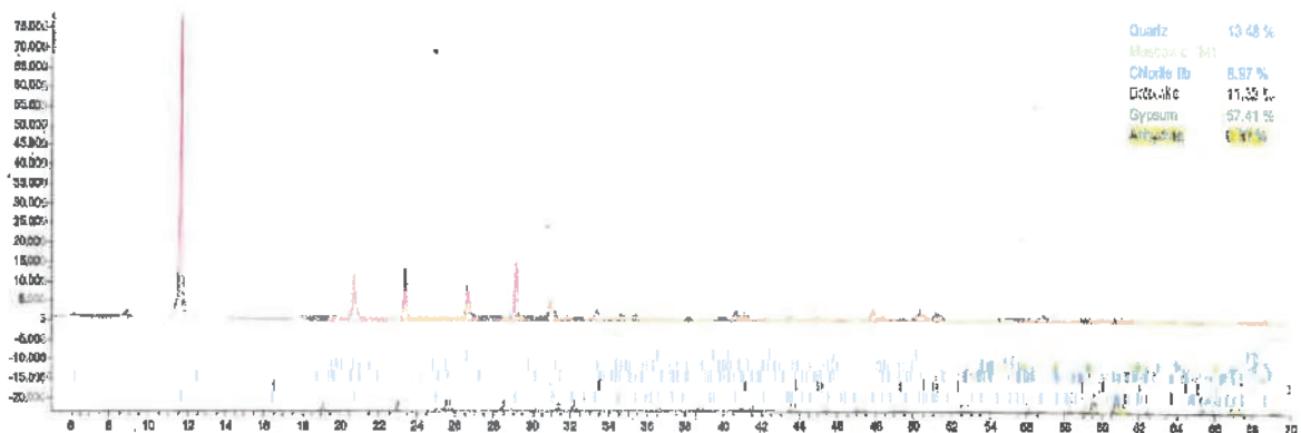
Abbildung 2: Auswertung und Schaubild der Probe B 3/24 – 60,4 m
