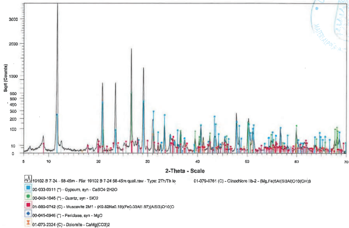
Abbildung 2: Schaubild der Probe B 7/24 – 58,45 m
