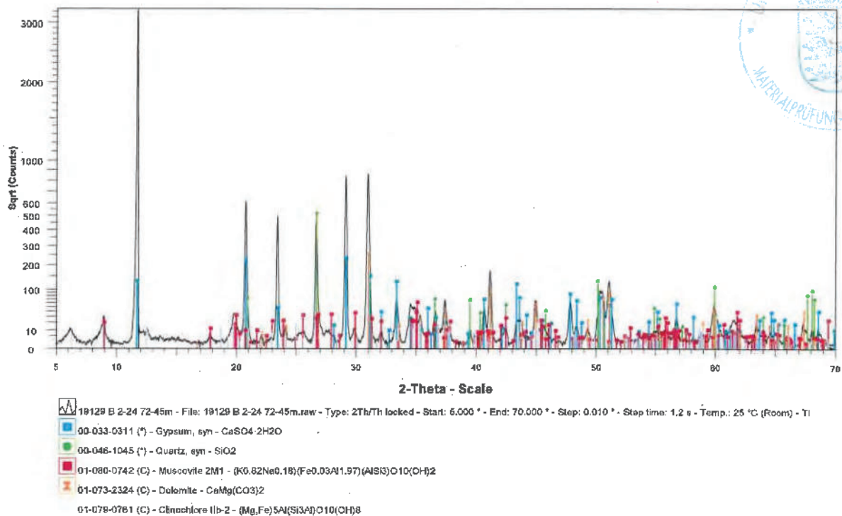
Abbildung 5: Schaubild der Probe B 2/24 – 72,45 m
