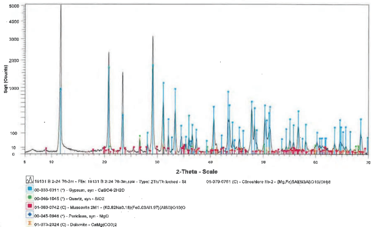
Abbildung 6: Schaubild der Probe B 2/24 – 76,30 m
