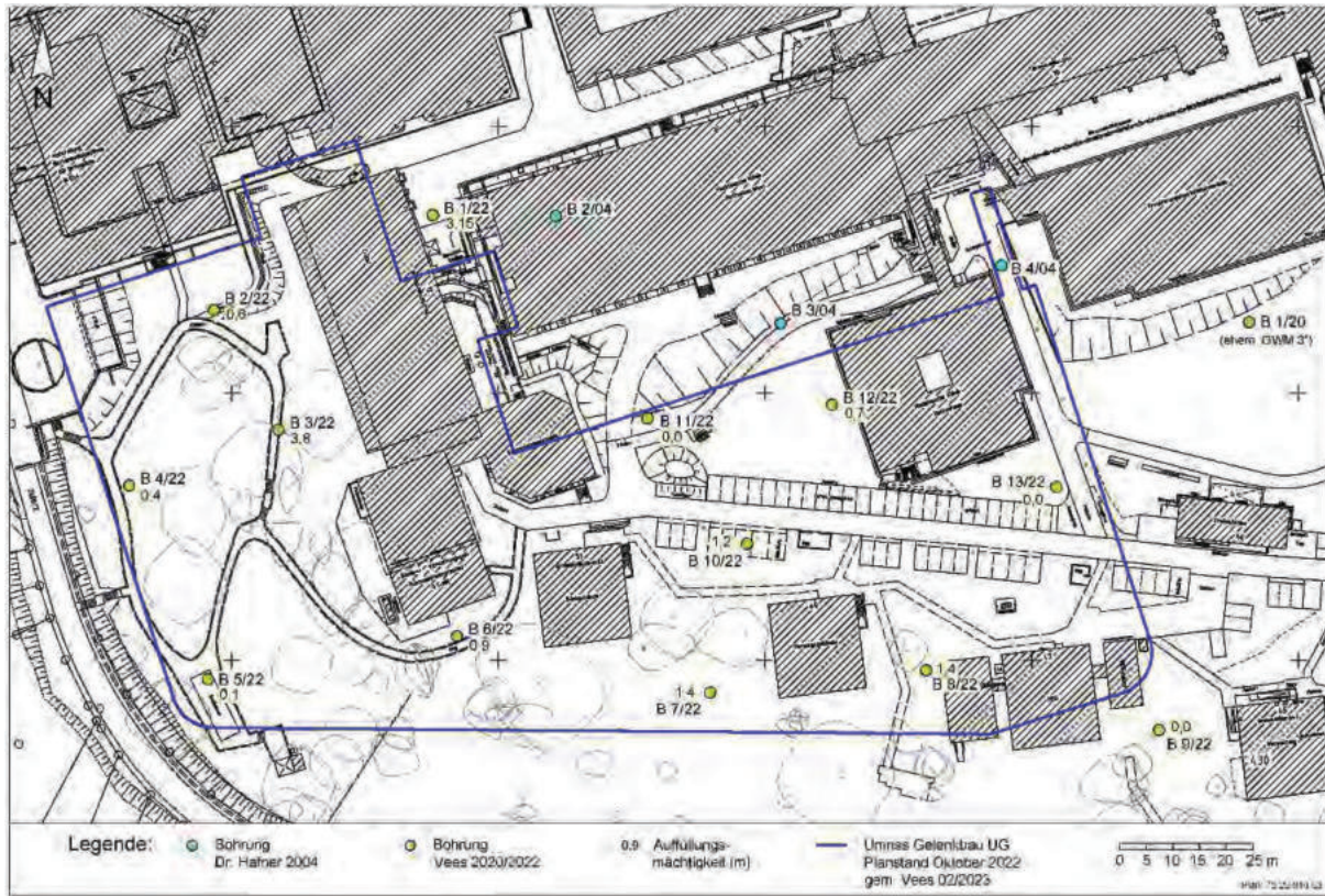
Abbildung 5: Lage der Bohrungen mit den festgestellten Auffüllungsmächtigkeiten
