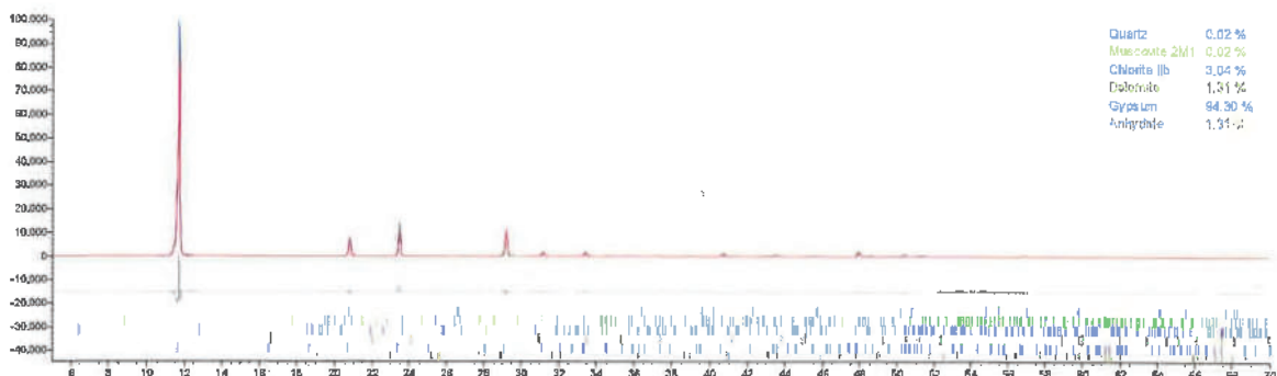
Abbildung 7: Auswertung und Schaubild der Probe 19107 B 7/24 – 64,6 m
