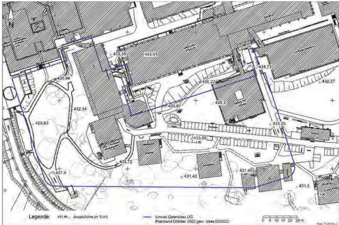
Abbildung 1: Übersichtslageplan mit Gebäudebestand und Geländehöhen (m TüH, Quelle: VEES/PARTNER)
