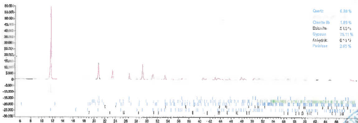
Abbildung 1: Auswertung und Schaubild der Probe B 3/24 – 58,8 m
